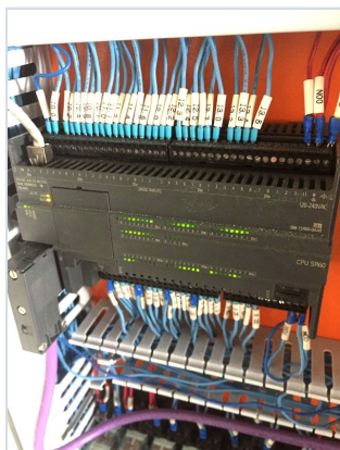
Lập trình & đấu nối PLC
