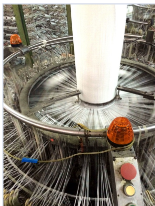
Cải tiến máy dệt
