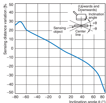
E3ZM-LS□2H(LS□7H)
