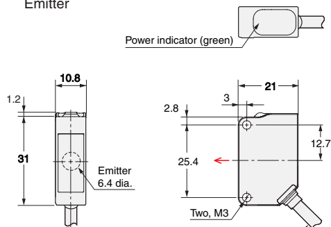
Emitter
