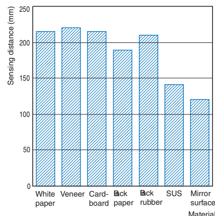
E3ZM-LS□4H(LS□9H)
