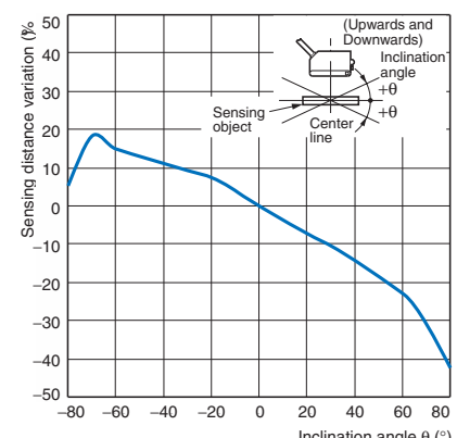
E3ZM-LS□4H(LS□9H)
