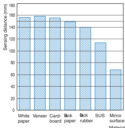
E3ZM-LS□2H(LS□7H)
