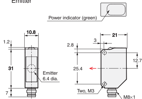
Emitter
